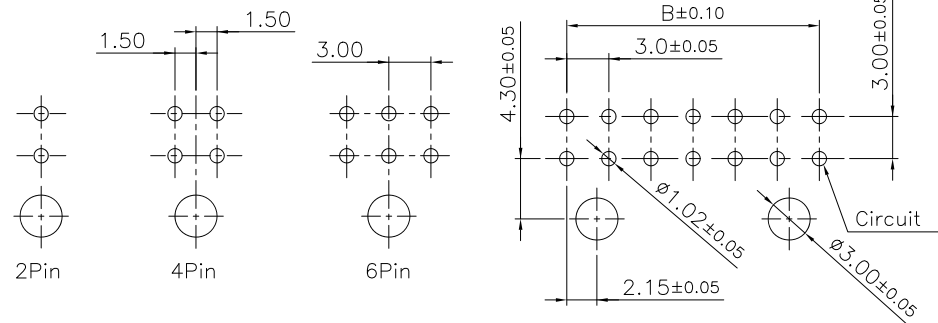
P.C.B. Layout
