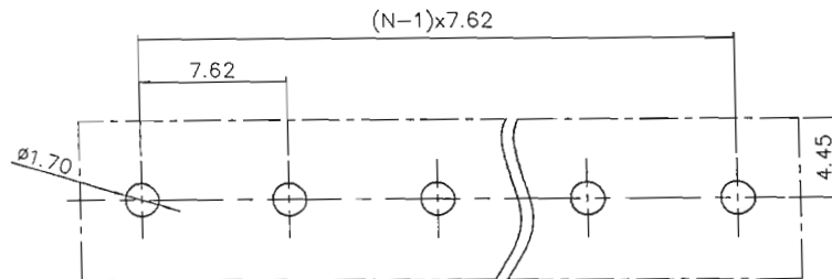
P.C.B LAYOUT
