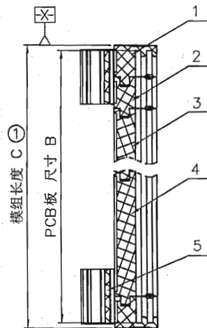
SEC A-A
