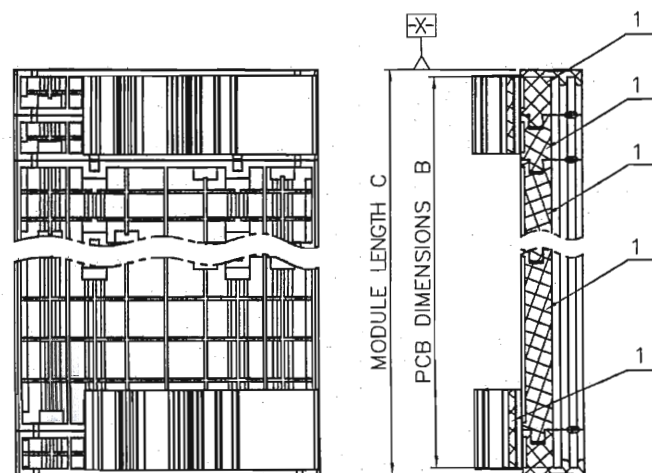
SEC A-A
