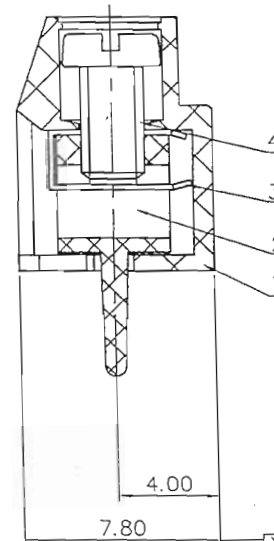
SEC A-A
