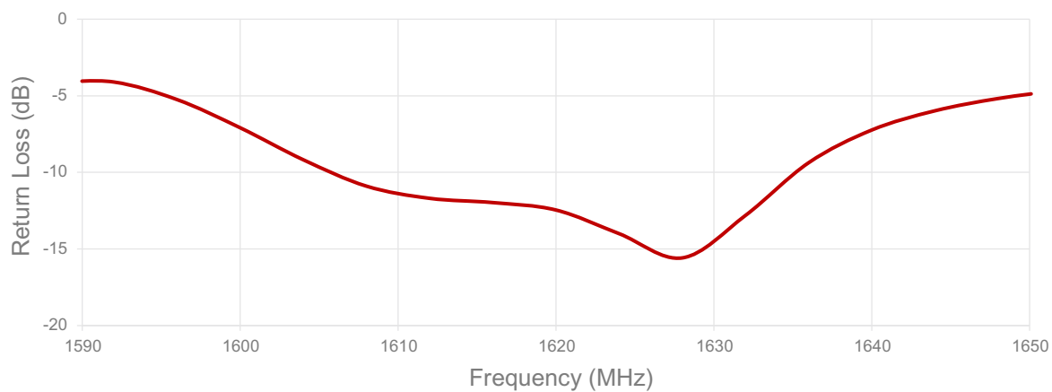
Cable 3: IRIDIUM
