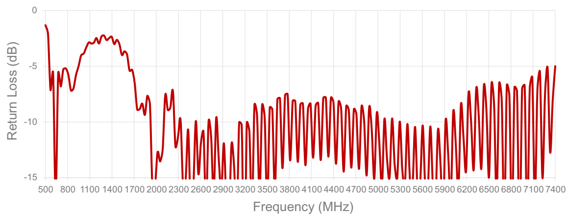
Cable 2: 5GNR
