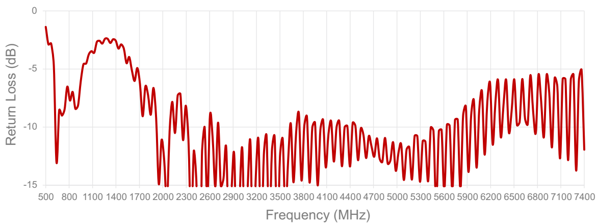
Cable 1: 5GNR
